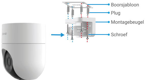
Afb. 1 Plafondmontage
