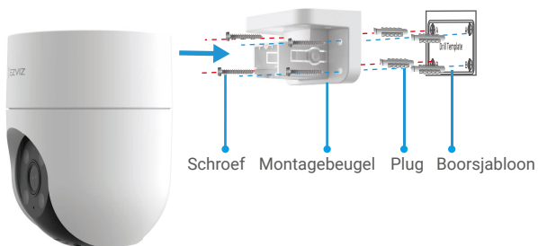
Afb. 2 Muurmontage
